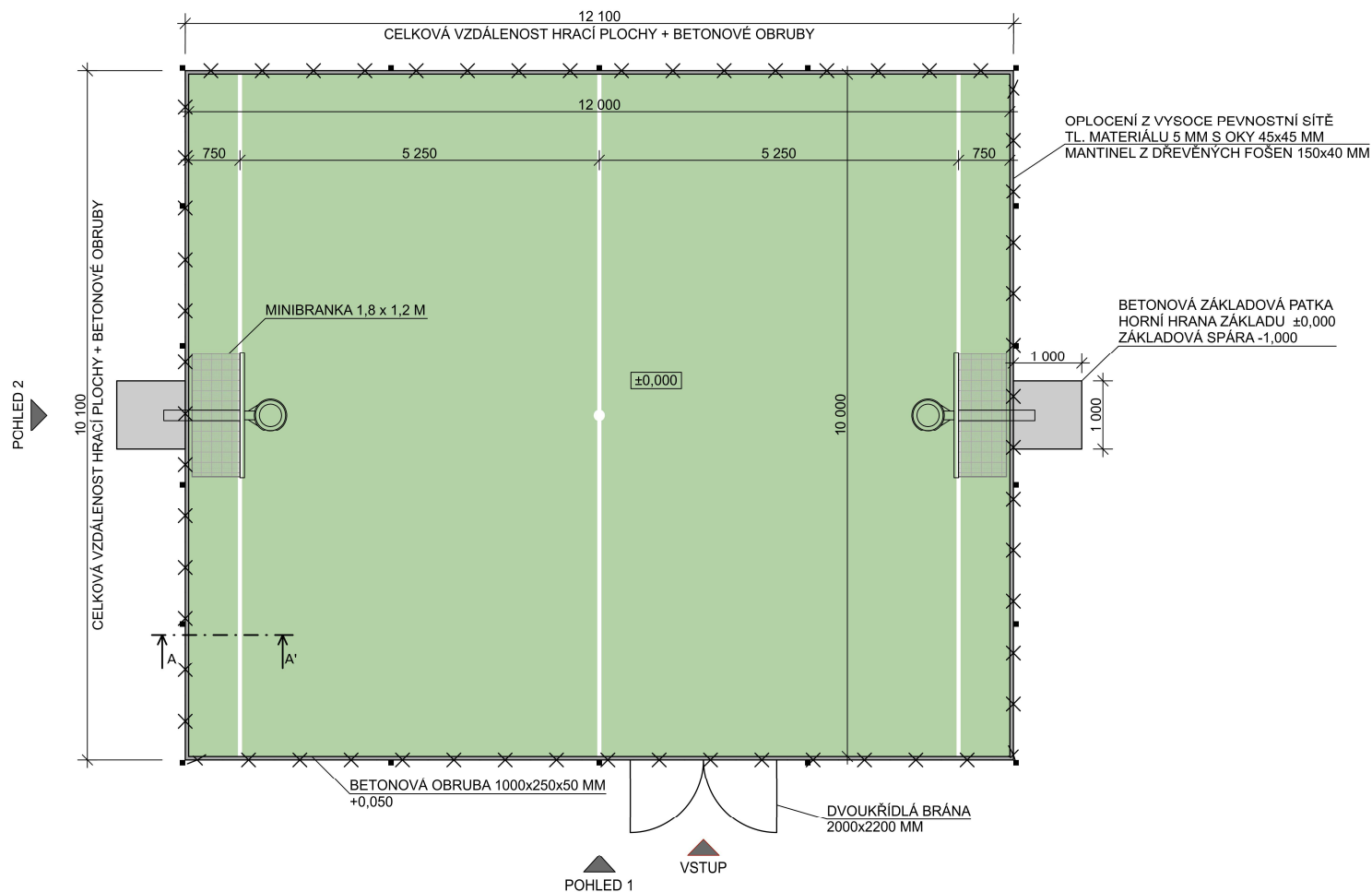
Obr. č. 2: Půdorys
